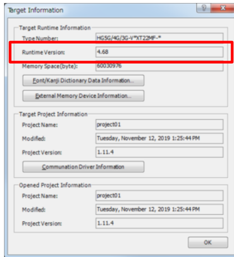
图-1：“系统信息”界面
