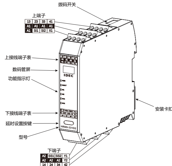
4-2. 系统模块图
