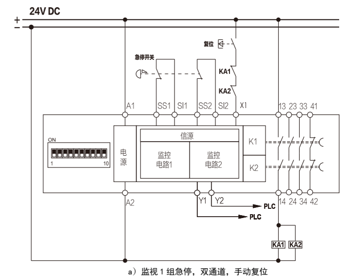
a) 监视 1 组急停，双通道，手动复位
