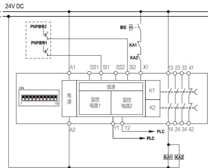
e) 监视 1 组 PNP 型安全光幕, 双通道, 手动复位
