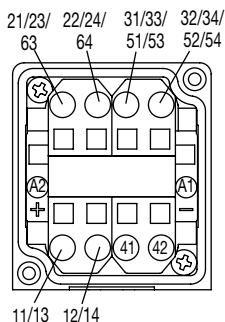
端子排列图
