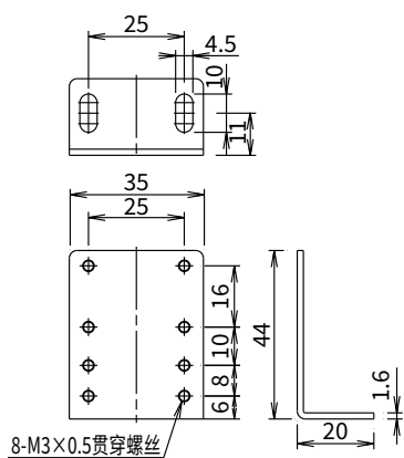
材质: SPCC
