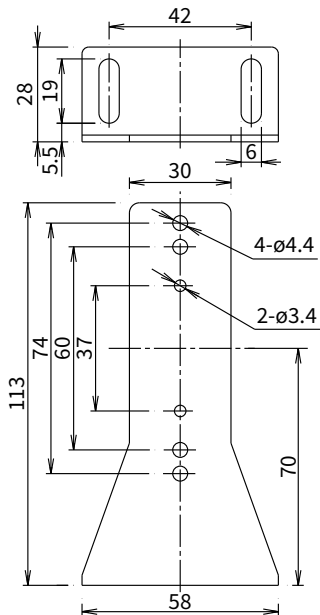
材质: SPCC
