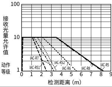
●接收光量—检测距离特性
