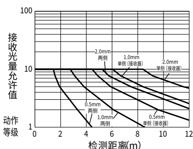
●平行移动特性(安装1.0mm垂直方向狭缝片时)
