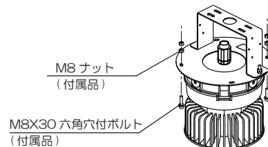
[天井取付金具使用時]
