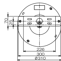
[天井取付金具使用時]
