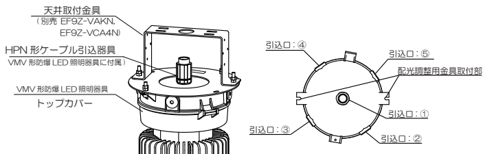
引込口配置図
