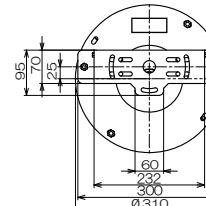
[角度調整取付金具使用時]
