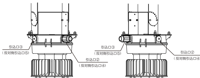
取付穴A使用時 例、引込口②使用
