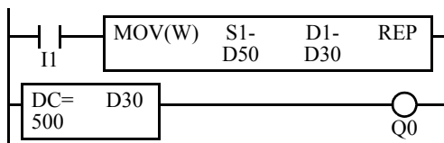
梯形图 2
