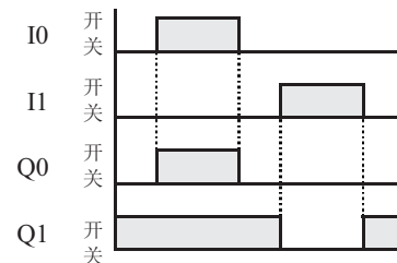
时序图
