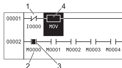
梯形图程序显示屏幕
