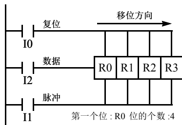
结构图
