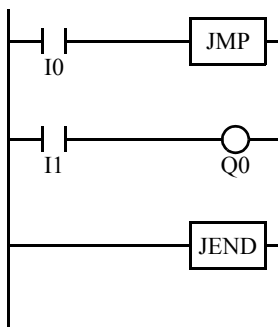
梯形图
