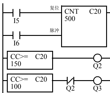
梯形图 4
