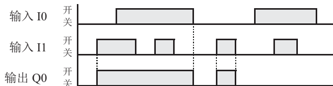
时序图
