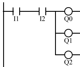
梯形图
