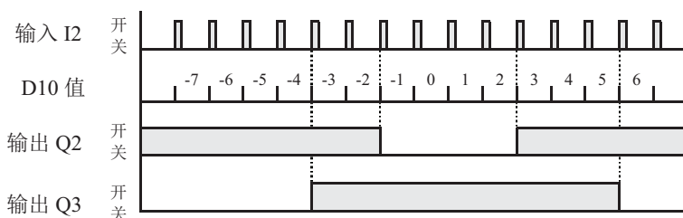
时序图
