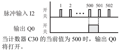
时序图
