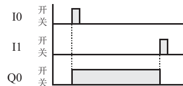
时序图
