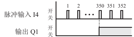
时序图
