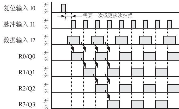
时序图
