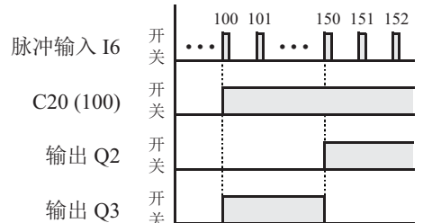
时序图
