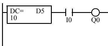
梯形图
