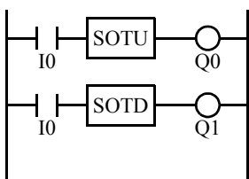
梯形图
